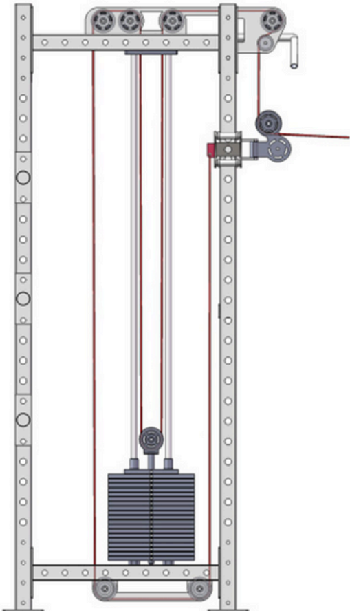
Diagrama de montaje del cable del entrenador:
